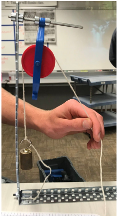
Fixed Pulley:
